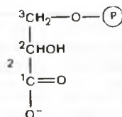
3-фосфоглицерат
