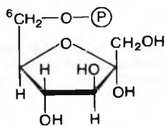
Фруктозо-6-фосфат
