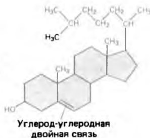
В. Стероид
