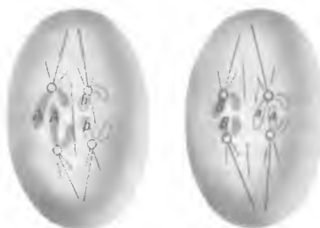
ТЕЛОФАЗА II
