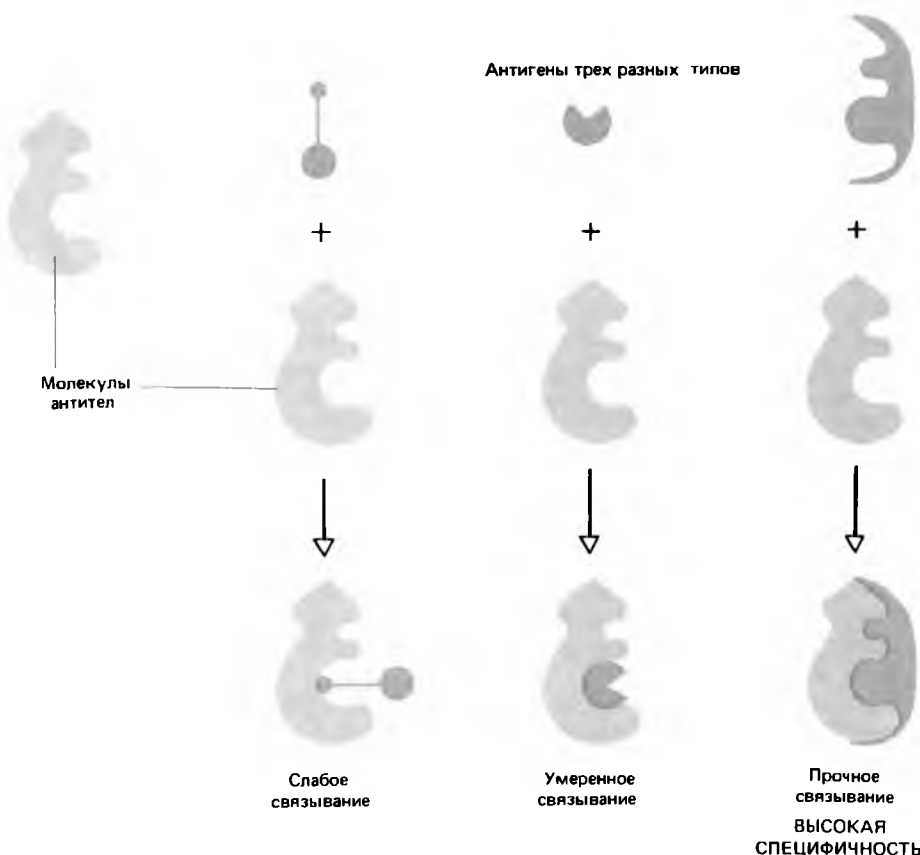
Рис. 22.11. Специфичность антител. Тип антител, схематически изображенный на рисунке, связывает антигены одного из трех типов гораздо лучше, чем антигены двух других типов. Ан-
