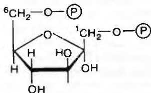
Фруктозо-1,6-бисфосфат
