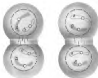
ТЕЛОФАЗА II
