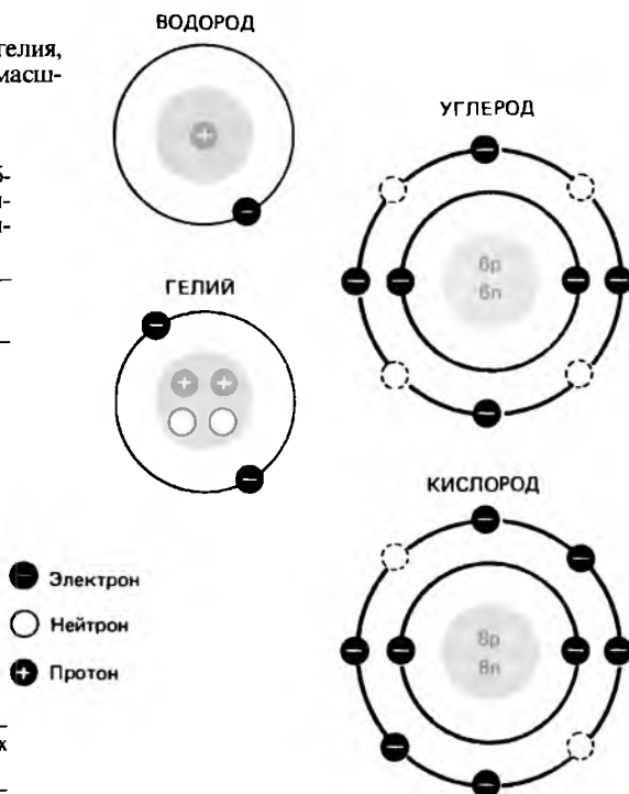
Рис. 9.3. Модели Бора для атомов углерода и кислорода (р – протон, n – нейтрон). Пунктирные кружки обозначают «пустые» области, которые могут заполняться электронами (разд. 9.2). На внешней оболочке атома углерода есть место еще для четырех электронов. Атом кислорода может присоединить еще два электрона, и тогда на его внешней оболочке их станет восемь, т.е. полный набор.
