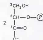
2-фосфоглицерат
