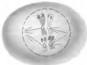
МЕТАФАЗА I
