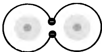
Модель Бора
