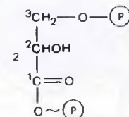
1,3-дифосфоглицерат
